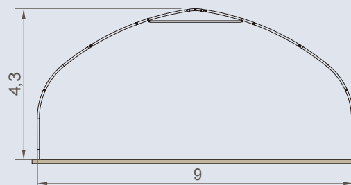
9 m - 1,5 m moduly
