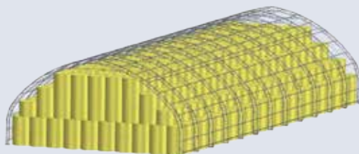
HALA 15 m - 41 balíků v řadě
